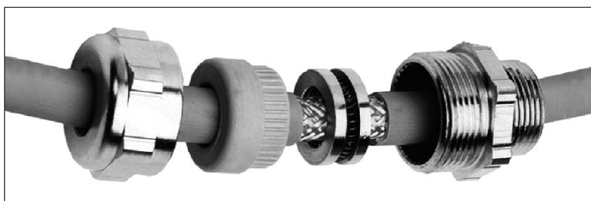
Bild 6: EMV-dichte Kabelverschraubung
