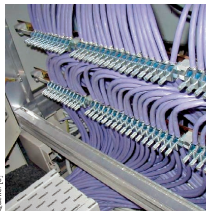
Bild 7: Kabelschirmklemmen am Verteilereintritt
